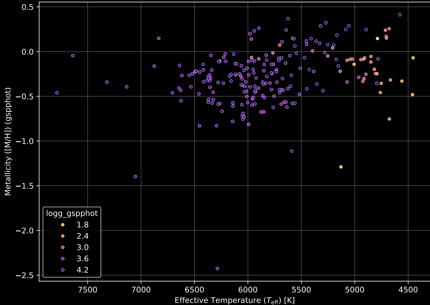
GALAH DR4 Field: [7186] Stellar Population Parameters (n= 218)
