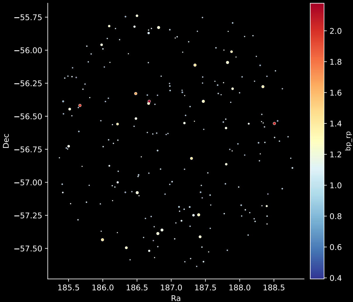
GALAH DR4 Field: [7186] Stars: 218
